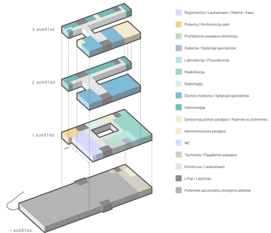
PASTATO FUNKCINĖ SCHEMA
